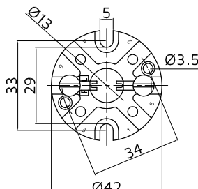
TBB600-AD
